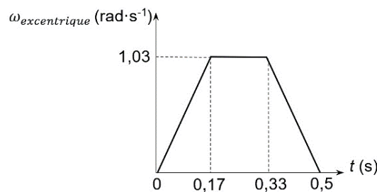
Figure 8 : loi de commande de vitesse de chaque excentrique (3)
