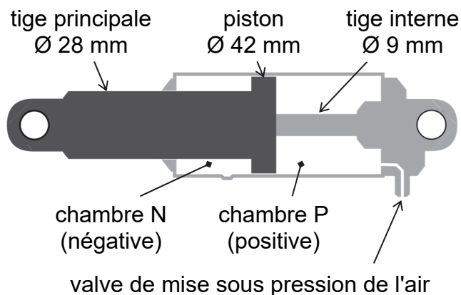
Figure 8 : ressort pneumatique
