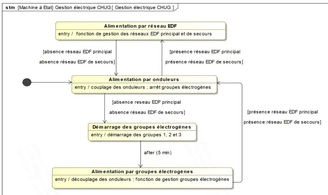
figure 6 : diagramme d'état incomplet de la gestion de l'alimentation électrique
