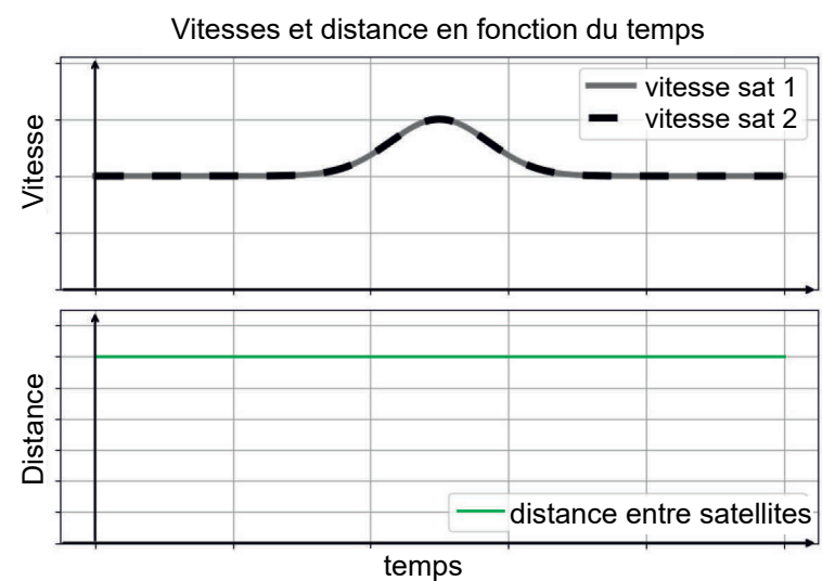
Figure 1. Propositions de représentation de l'évolution de la vitesse des satellites et de leur distance relative lors du passage au-dessus de l'objet massif
